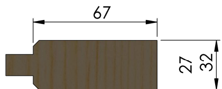
Emboîture 68 mm 27 ou 32 (2)
