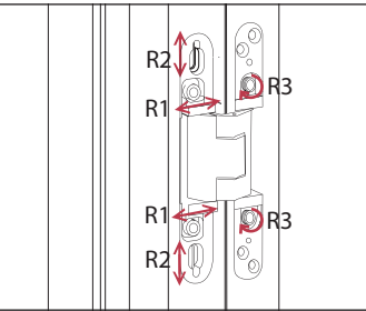
Ajustement horizontal, vertical et aplomb de la porte.
