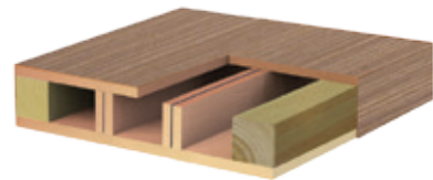
Panneaux et renforts intérieur, MDF haute résistance. Panels and internal reinforcements, MDF high strength.
