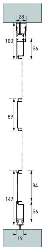
Coupe vue de profil
