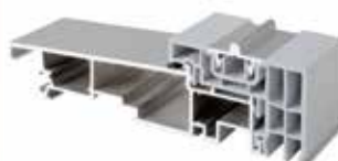
Seuil alu à rupture thermique
