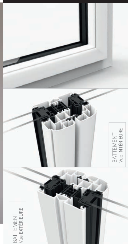
Fenêtre en bicoloration présentée avec poignée ALFA.
